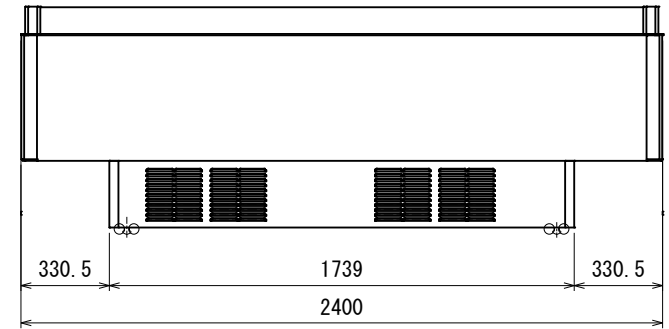
(S=1:20)
