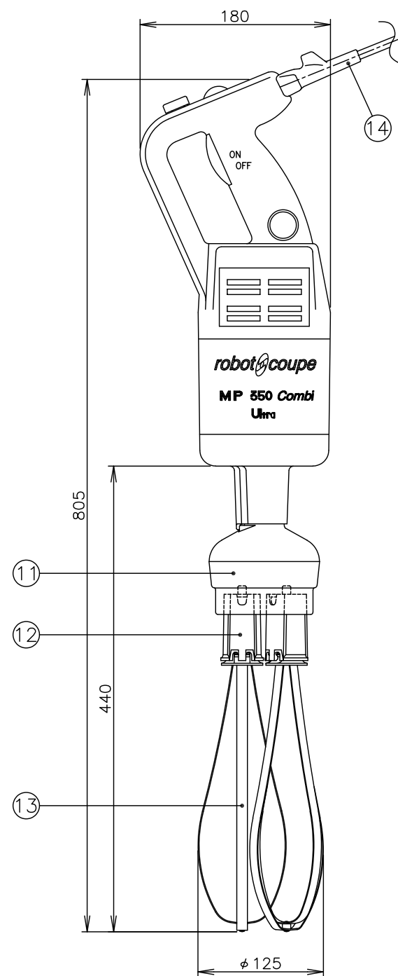
ホイッパー装着図
