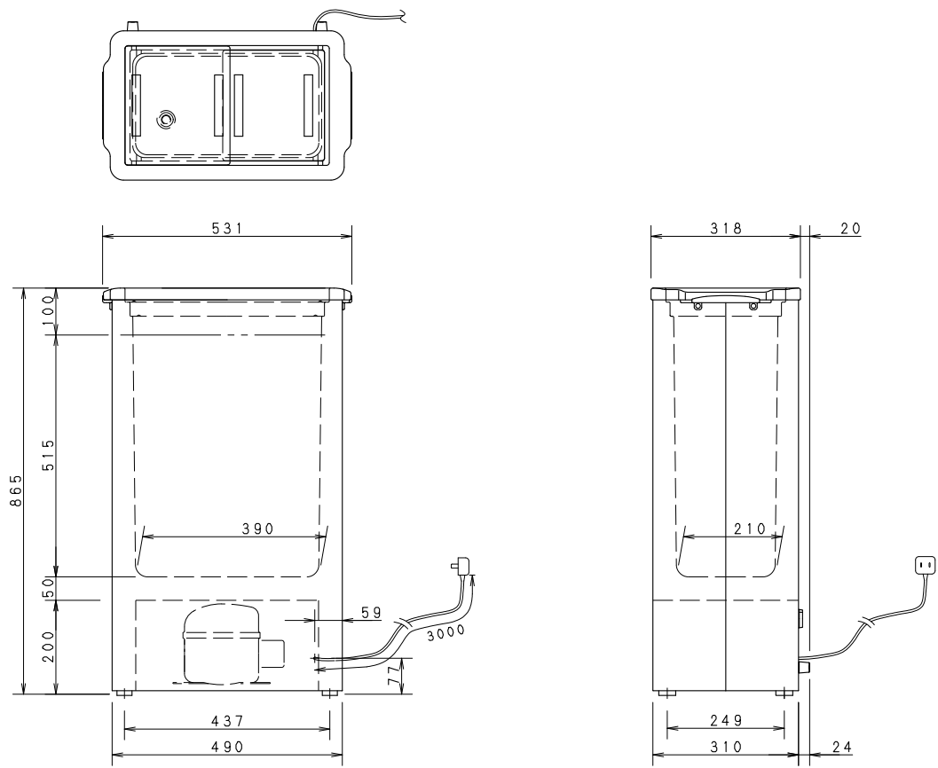
キャスター取付位置 (台脚裏側)
