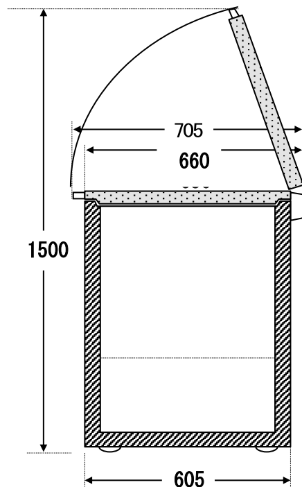
側面
