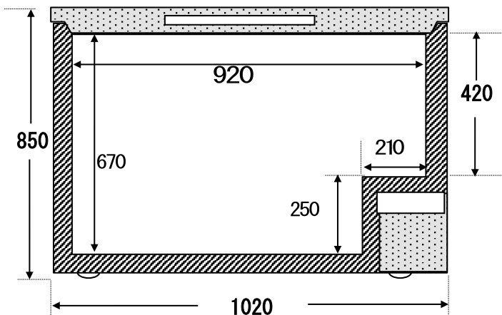
正面
